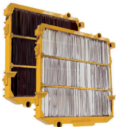
Охлаждение ДВС со съемными трубками
